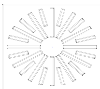
RBN-P2 jelű réselrendezés (örvényes 2 soros)
